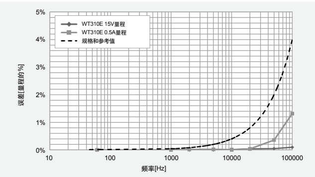
共模电压对读数影响 (输入600Vrms共模电压时)
