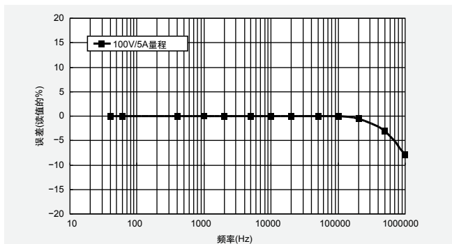
频率-功率精度特性曲线示例
