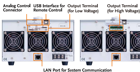
后面板
