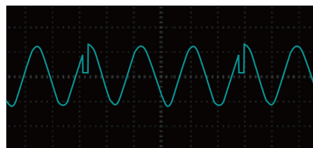
陷波波形
