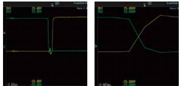
变频器门极信号波形(20kHz)
