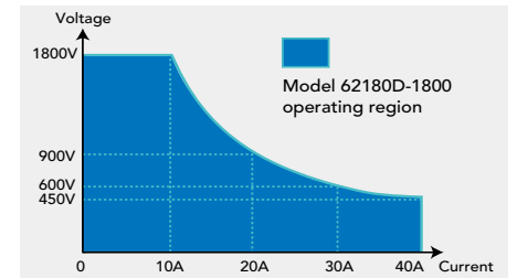
62180D-1800操作范围(Source Mode)
