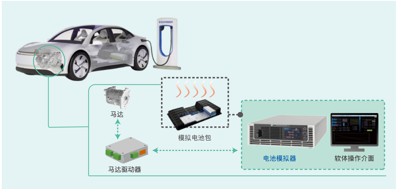
汽车启停系统马达驱动器测试应用
